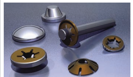
STARLOCK Lock washer טבעת נעילה
